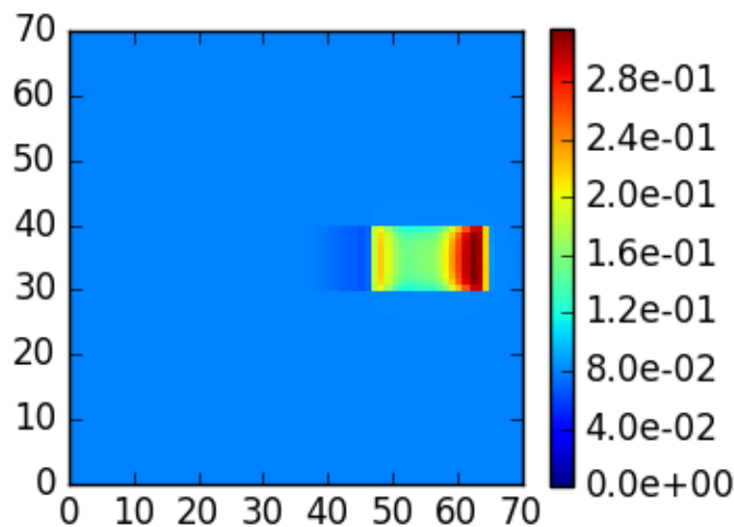
mcart_fmc case 4, \theta_0=20 , z=0 , \theta=40 , \phi=180
