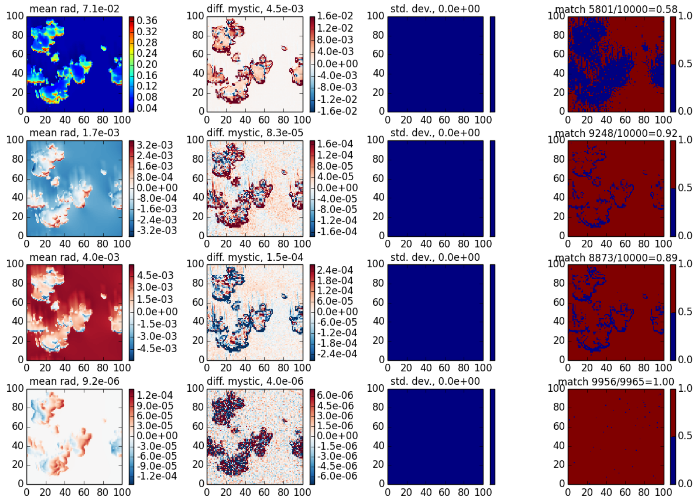
shdom3 case 3, \theta_0=20 , z=0 , \theta=40 , \phi=120
