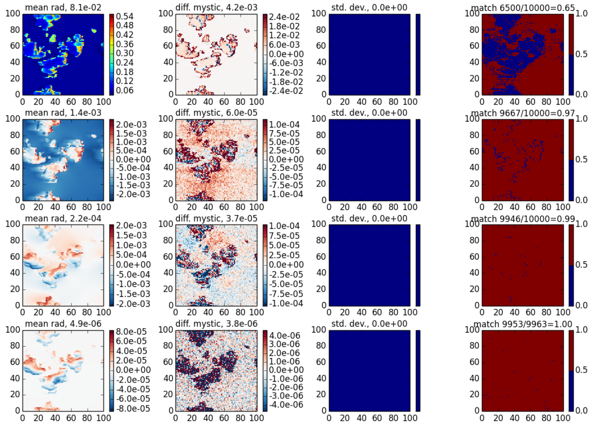
shdom3 case 4, \theta_0=20 , z=0 , \theta=40 , \phi=180
