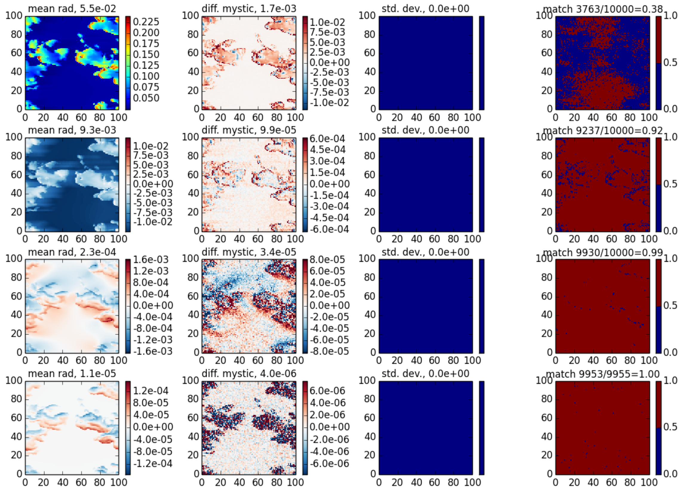
shdom3 case 1, \theta_0=20 , z=0 , \theta=40 , \phi=0
