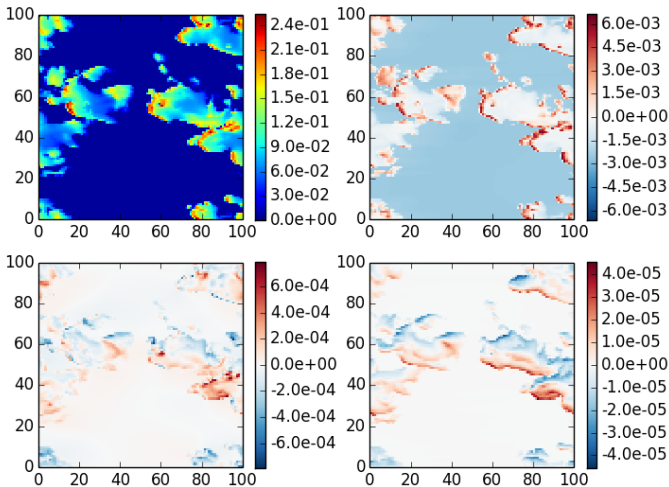
shdom3 case 1, \theta_0=20 , z=0 , \theta=40 , \phi=0
