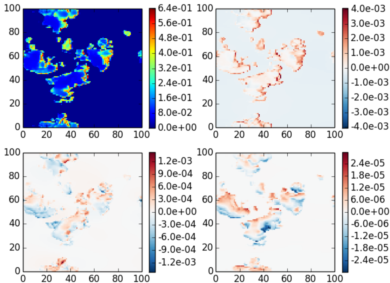
shdom3 case 4, \theta_0=20 , z=0 , \theta=40 , \phi=180
