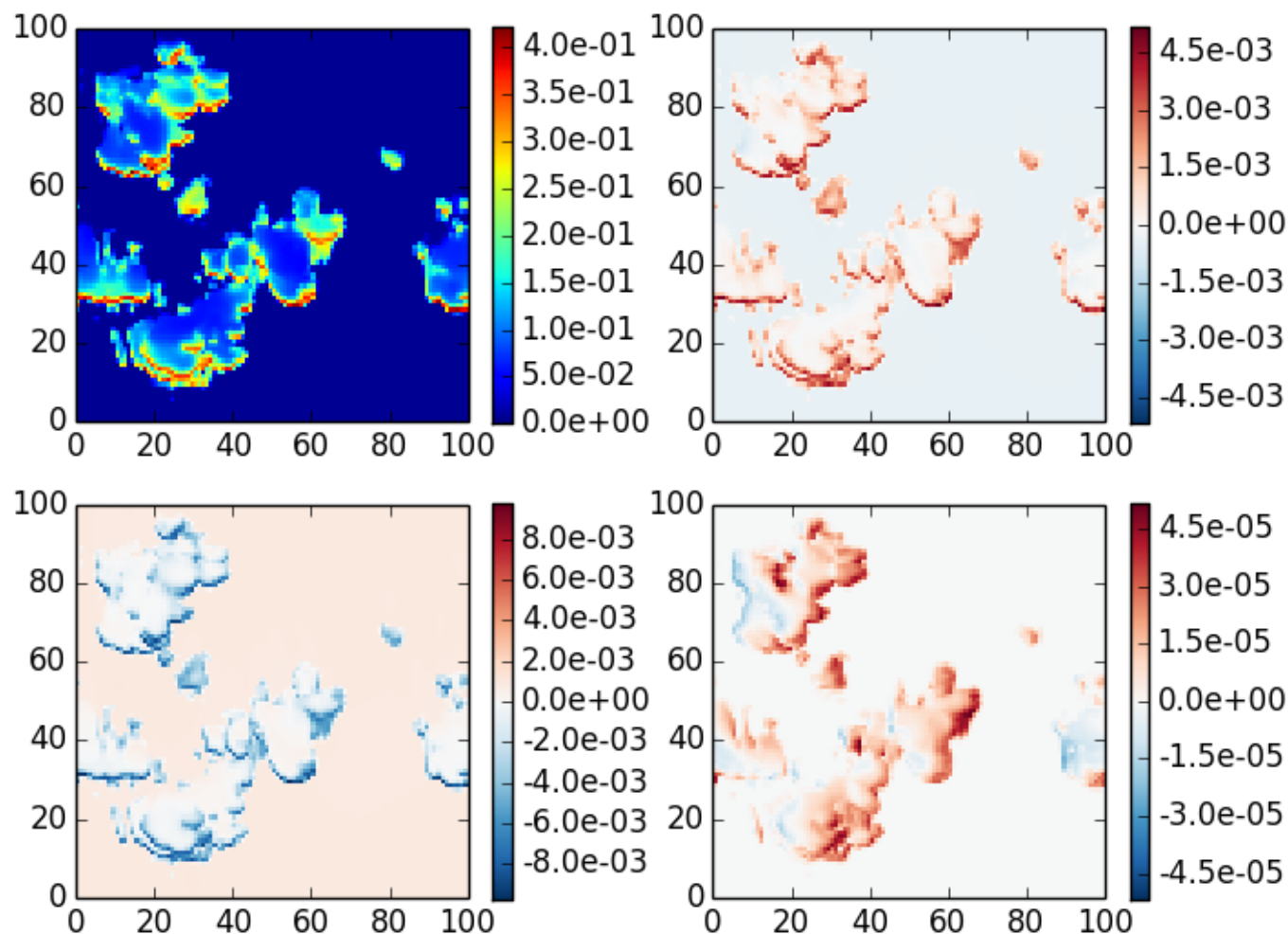
shdom3 case 3, \theta_0=20 , z=0 , \theta=40 , \phi=120
