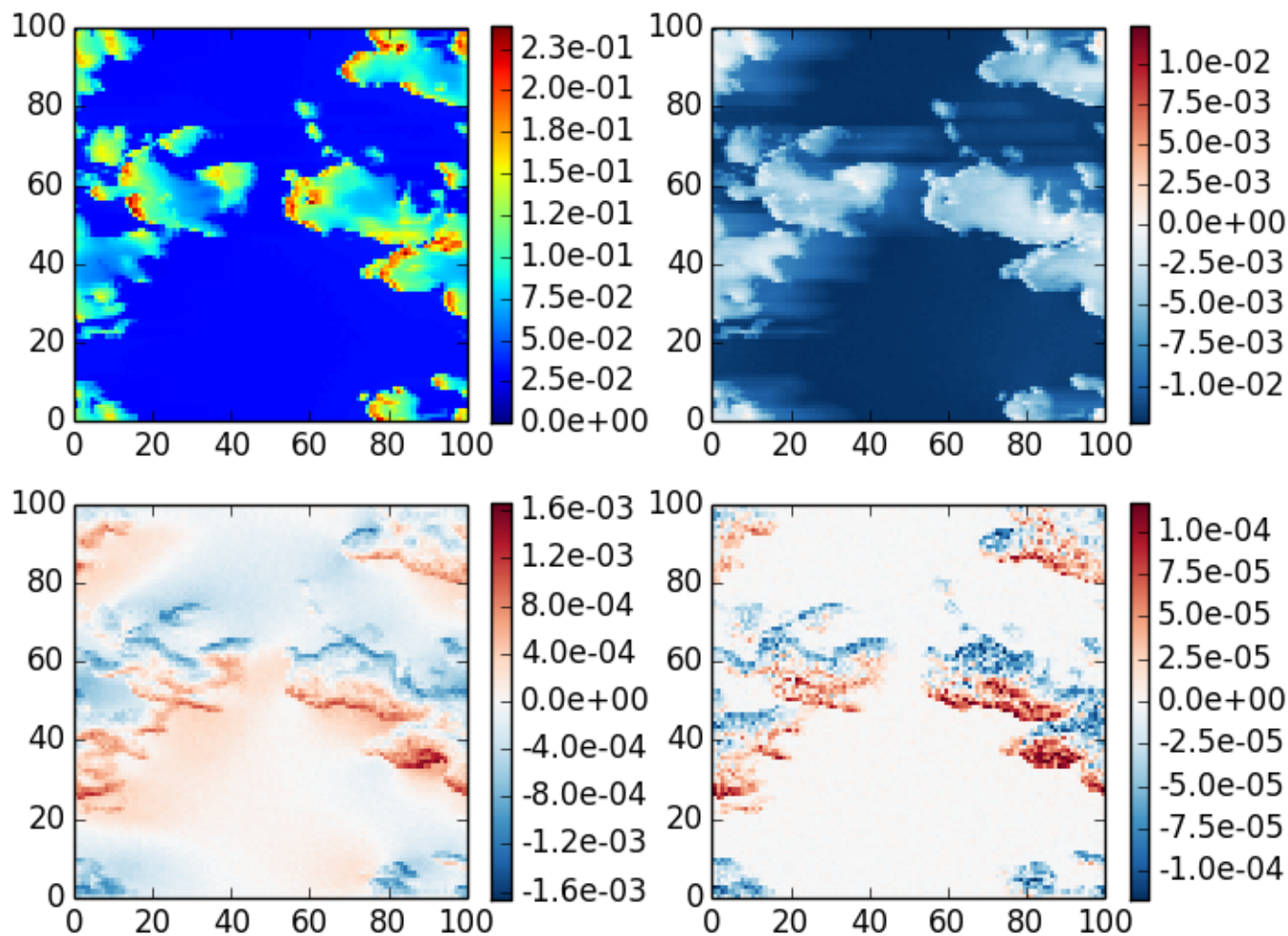
mscart_fm case 1, \theta_0=20 , z=0 , \theta=40 , \phi=0
