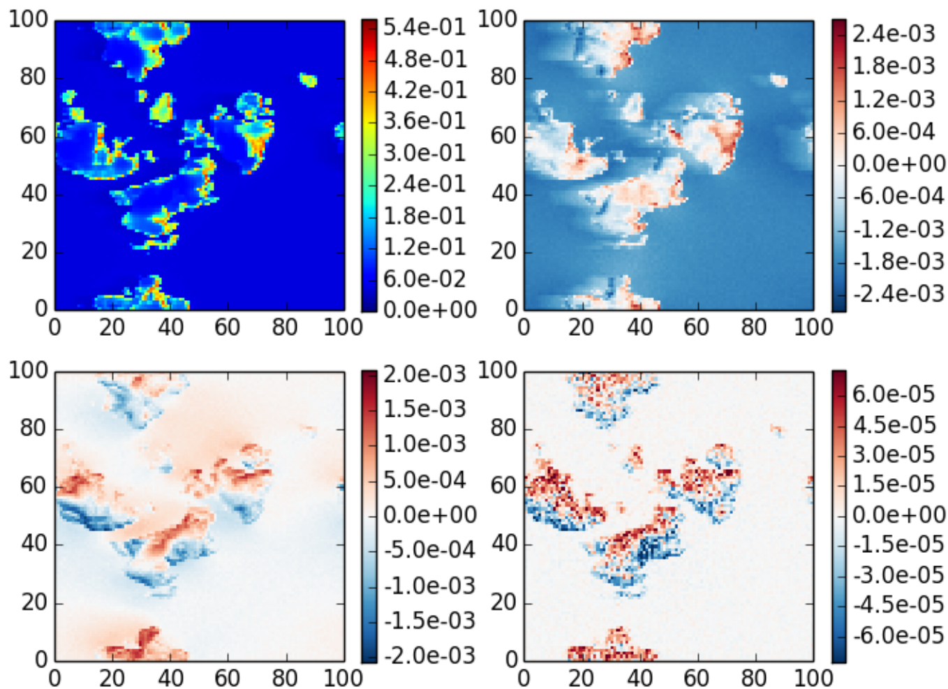
mscart_fm case 4, \theta_0=20 , z=0 , \theta=40 , \phi=180
