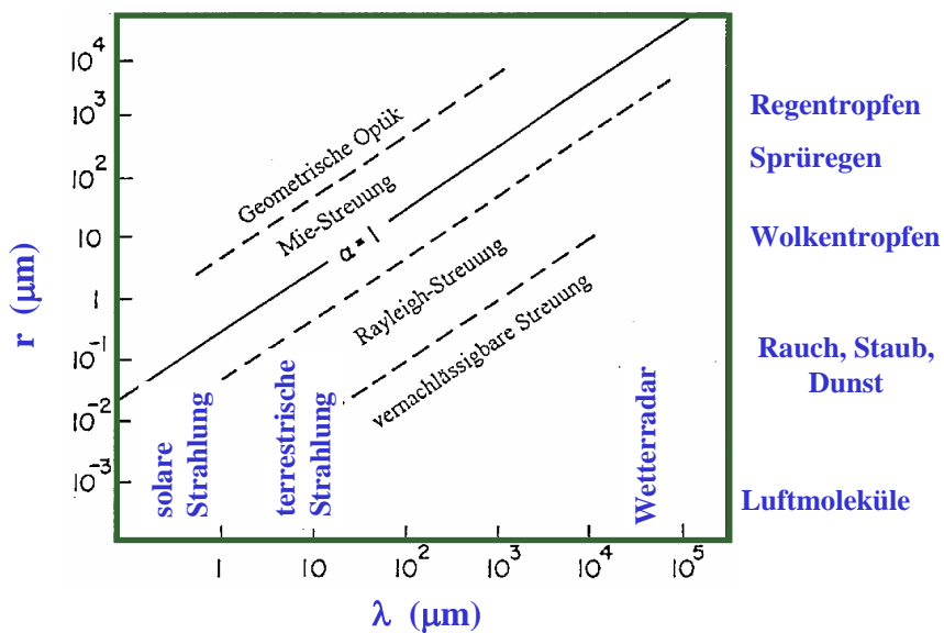
Der Größenparameter in Abhängigkeit von der Wellenlänge \lambda und dem Teilchenradius r .
